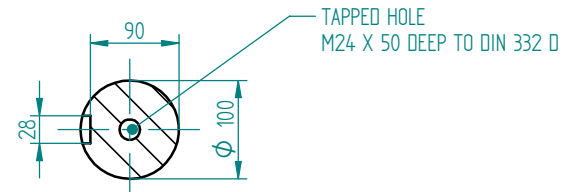
Przekrój A-A 1:5
