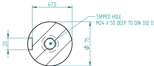
Przekrój A-A 1:2
