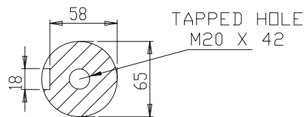
SECTION A-A SCALE 1 : 3
