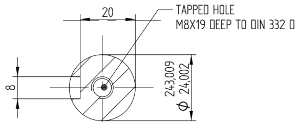
Przekrój A-A 1:1
