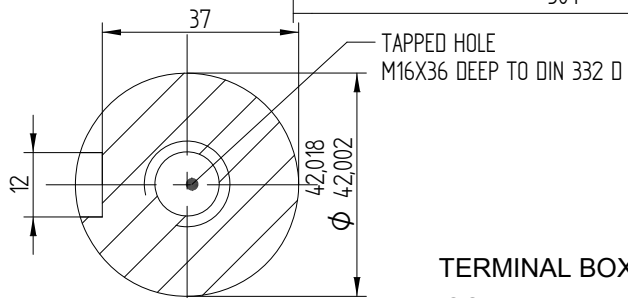
Przekrój A-A 1:1
